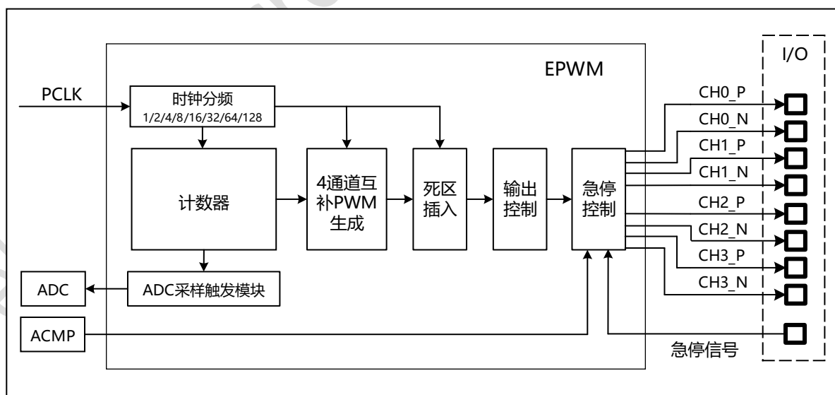
图 13-1 EPWM 模块结构框图
