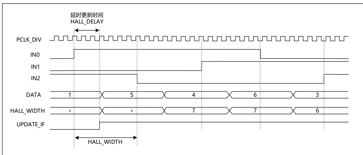
图 14-5 霍尔输入模式示意
