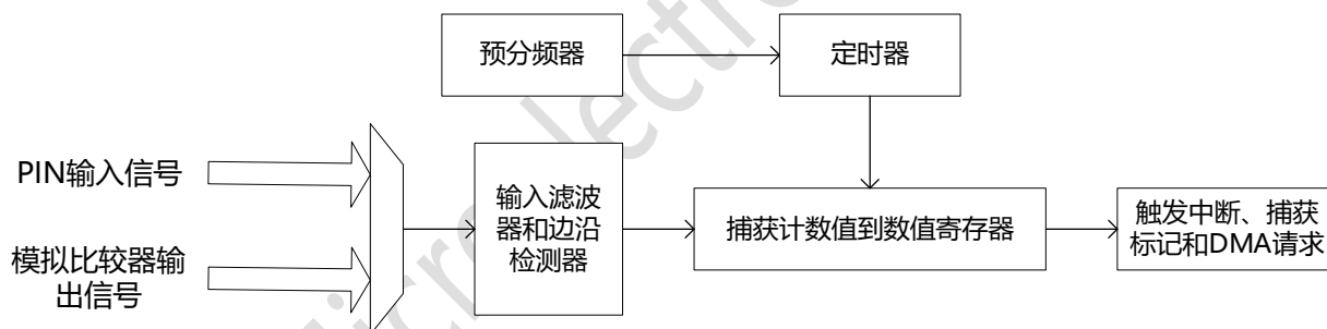
图 12-1 捕获模式
