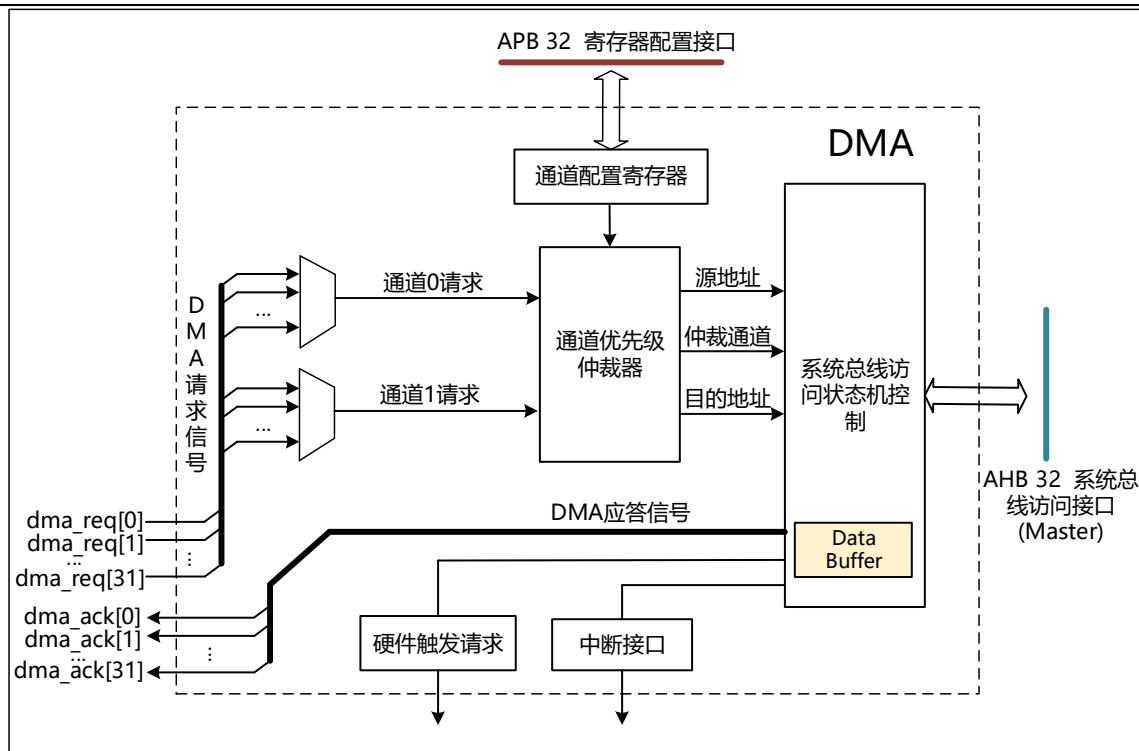
图 8-1 DMA 框图
