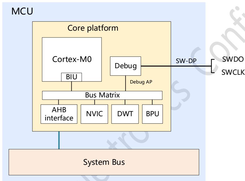
图 28-1 DPM32 MCU 和 Cortex®-M0 调试支持框图
