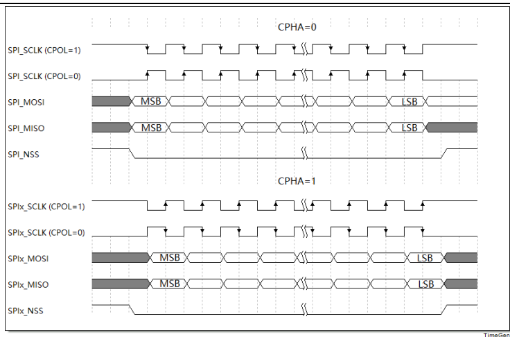
图 20-5 SPI 传输数据时序图
