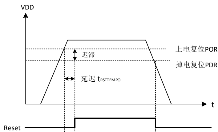
图 4-1 POR 与 PDR 复位的时序关系
