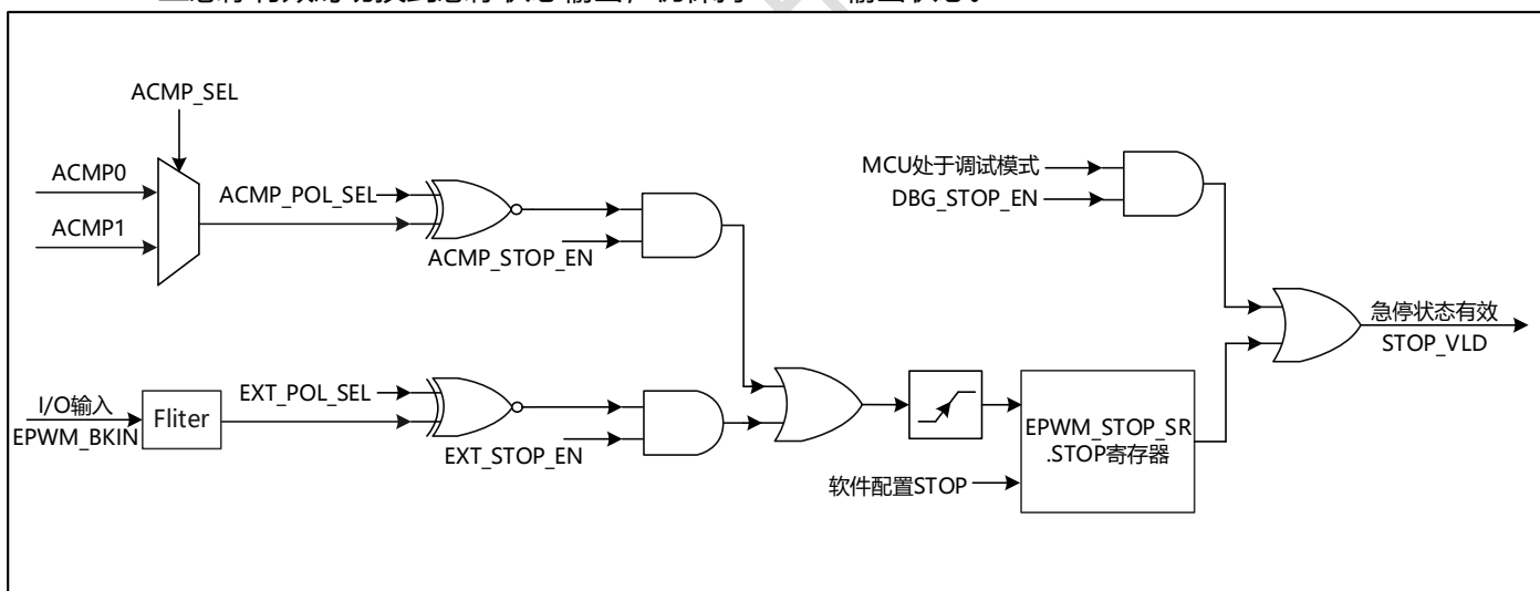
图 12-5 急停控制模块
