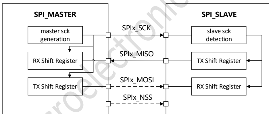
图 18-3 SPI 单工引脚连接图
