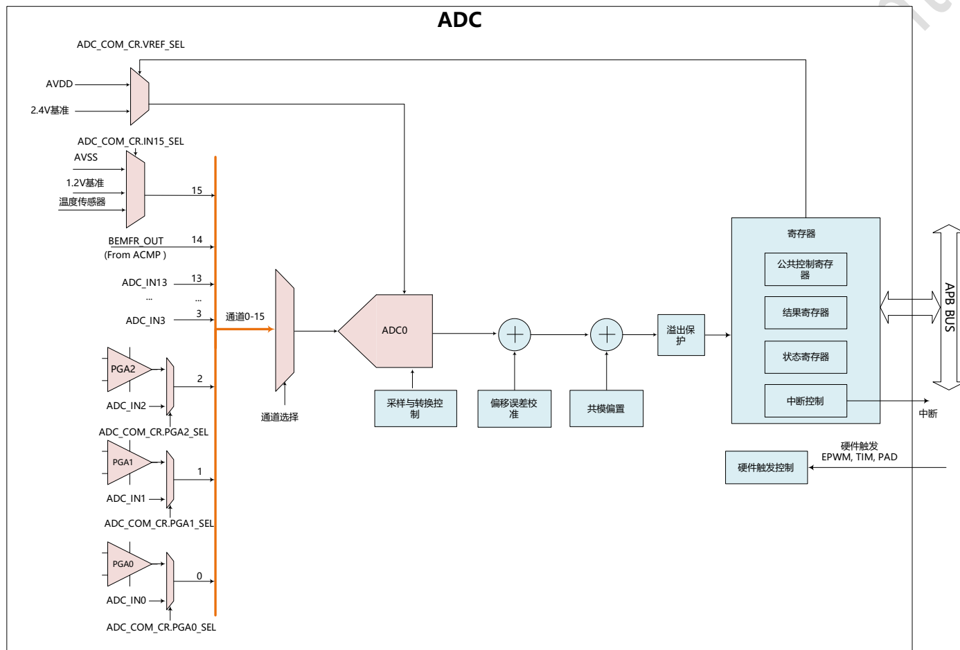
图 20-1 ADC 模块结构框图
