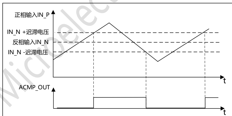
图 22-2 比较器迟滞
