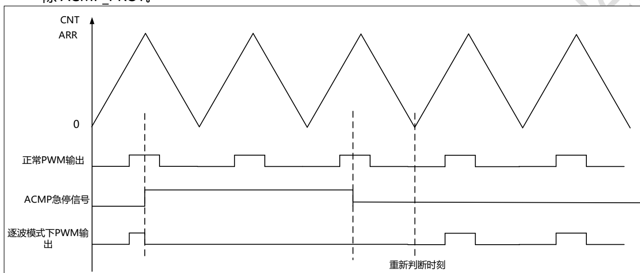
图 12-6 ACMP 逐波模式
