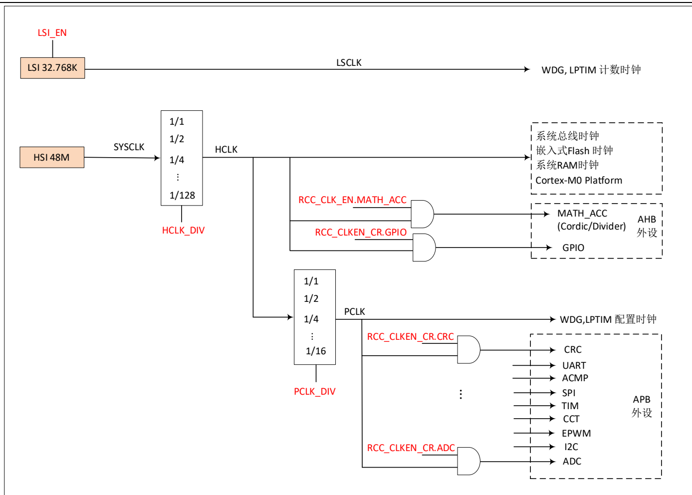
图 5-1 RCC 时钟树框图
