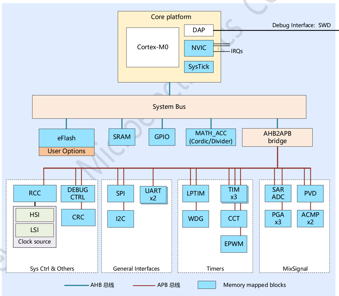
图 2-1 系统架构
