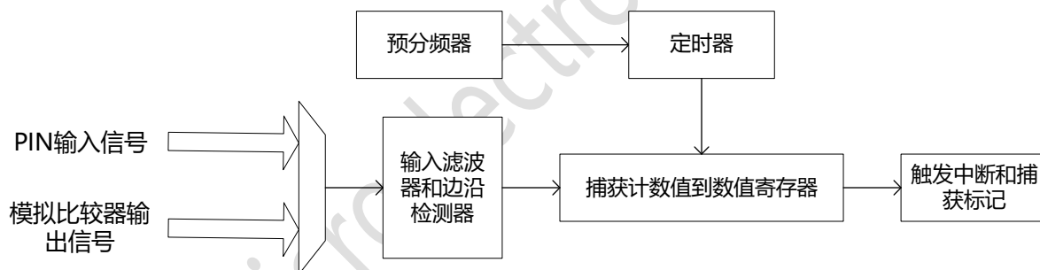
图 11-1 捕获模式
