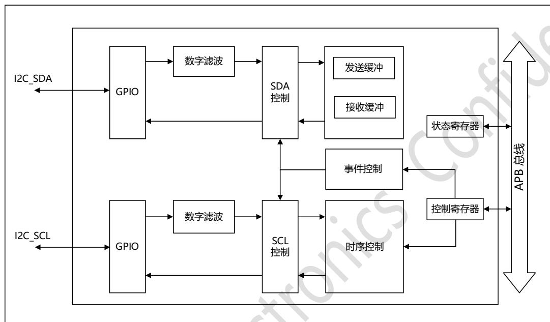
图 16-6 I2C 模块结构框图
