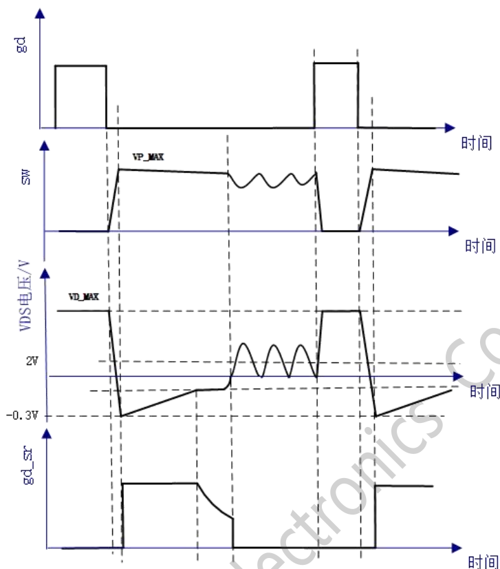
功能波形图
